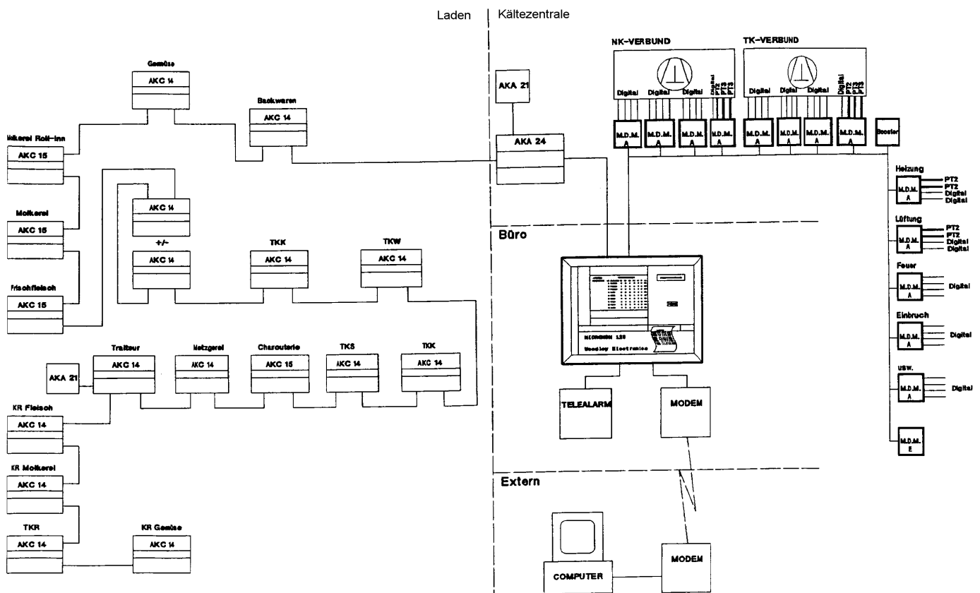
Bild 3: Systemeinbindung Kälte und Haustechnik
