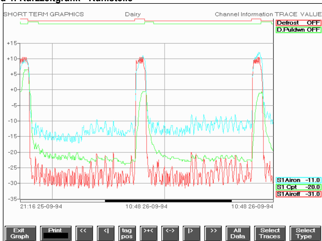
Bild 4: Kurzzeitgrafik - Kühlstelle
