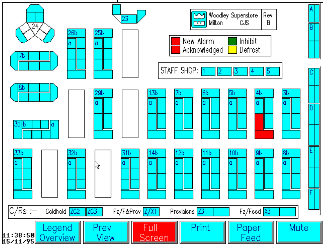
Bild 3: Übersichtsseite Supermarkt
